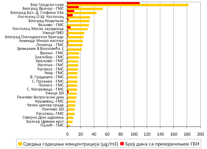
Упоредни приказ средње годишње концентрације сумпордиоксида ( \mu\text{g}/\text{m}^3 ) у амбијенталном ваздуху и броја дана са прекорачењем ГВИ за изабрана места у 2007. години
