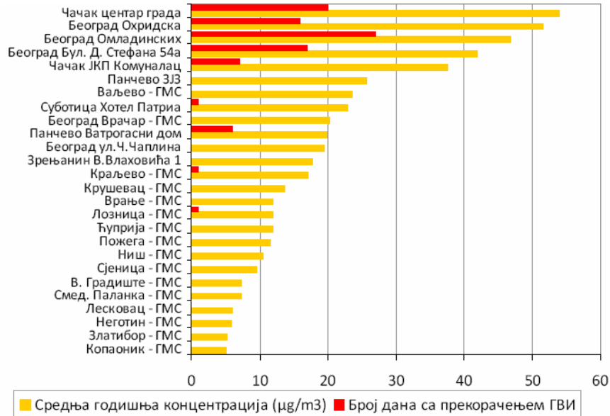
Упоредни приказ средње годишње концентрације азотдиоксида ( \mu\text{g}/\text{m}^3 ) у амбијенталном ваздуху и броја дана са прекорачењем ГВИ за изабрана места у 2007. години
